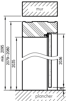
COUPE VERTICALE OP POUR PORTES VITRÉES
