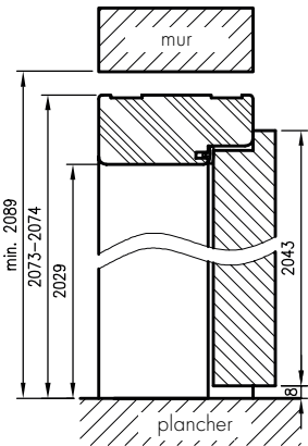
COUPE VERTICALE OP POUR PORTES À RECOUVREMENT
