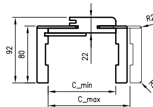
Coupe ORB 095-300
