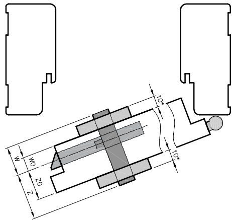
Dessin Choix des dimensions du cylindre
