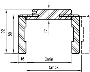
Coupe OR avec cornière. T80
