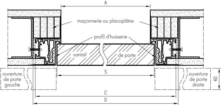
Coupe transversale de la porte Sara Eco2 à chant droit - ouverture vers l'extérieur
