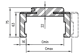
Coupe OR/ORC avec cornière. T63
