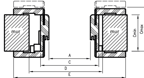
Coupe horizontale ORB
