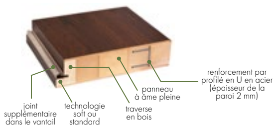
COUPE TRANSVERSALE DU VANTAIL DE PORTE HERSE 32 dB
