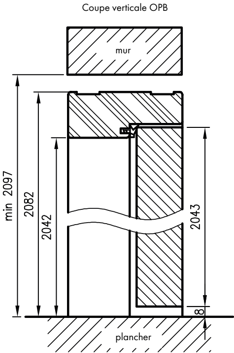
Pour porte simple vantail
