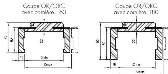
Coupe horizontale OR/ORC
