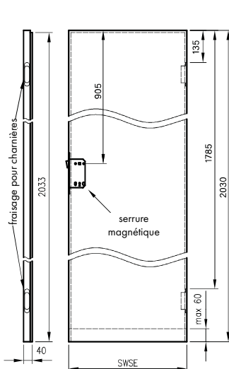
Vantaux Sara Eco 2 à recouvrement selon la norme 202X
