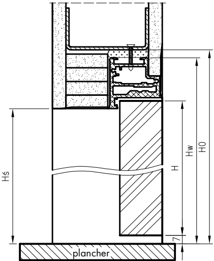
Coupe verticale de la porte Sara Eco 2 à chant droit - ouverture vers l'extérieur
