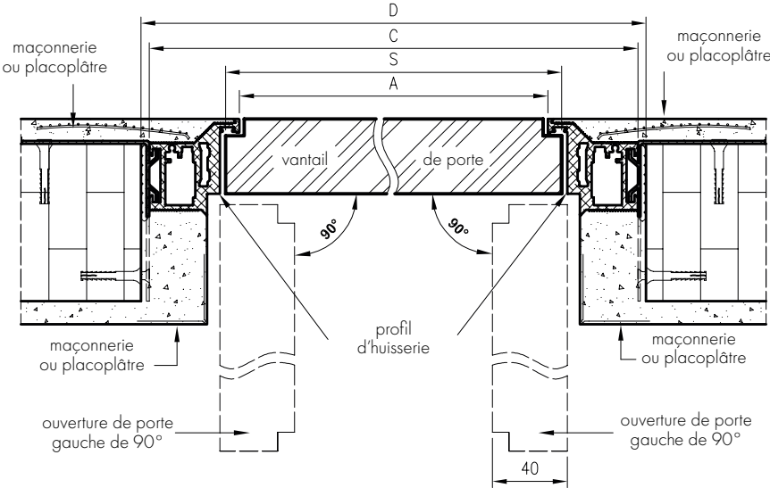
Coupe transversale de la porte Sara Eco2 à recouvrement – ouverture vers l'intérieur
