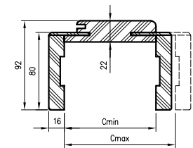
Coupe OR/ORC avec cornière. T80
