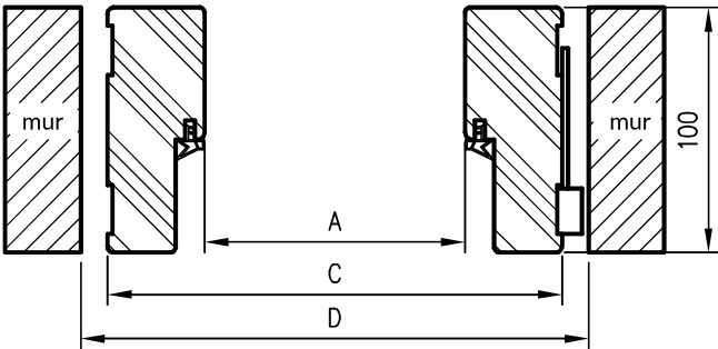
Coupe horizontale OPB
