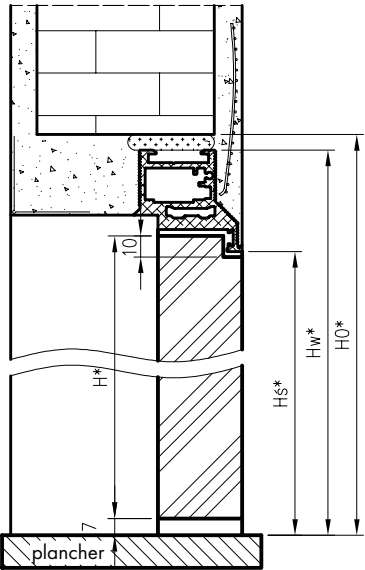
Coupe transversale de la porte Sara Eco2 à recouvrement – ouverture vers l'intérieur
