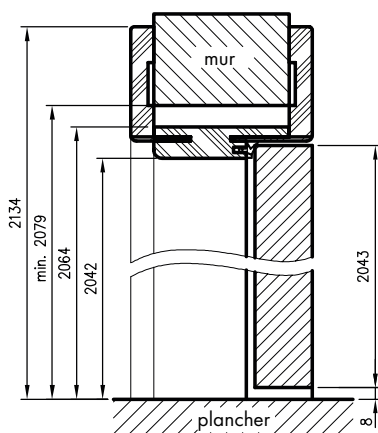
Coupe verticale de porte à chant droit ORB
