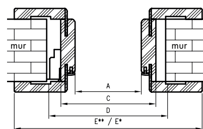
Coupe horizontale OR/ORC
