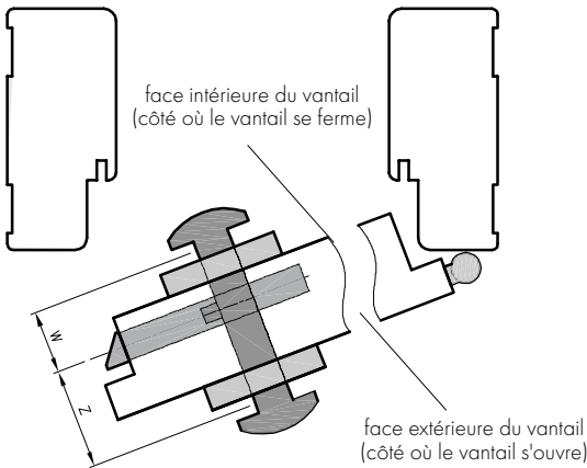
Dessin Choix des dimensions du cylindre avec bouton moleté
