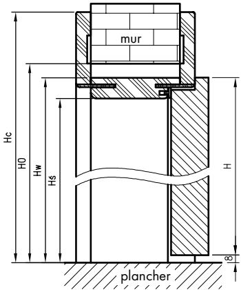
Coupe verticale OR
