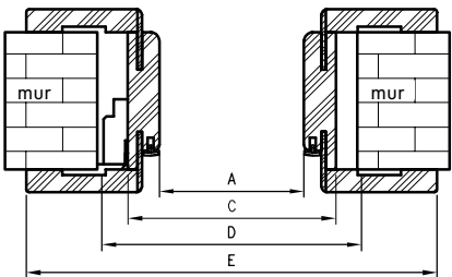
Coupe horizontale OR
