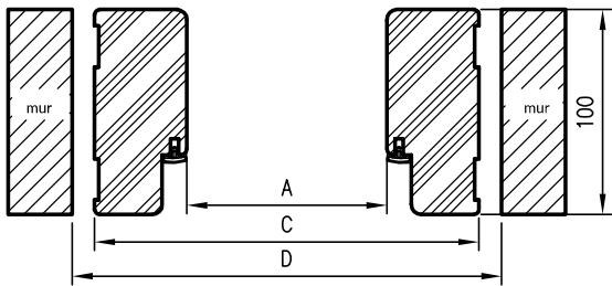
Dimensions pour porte simple vantail
