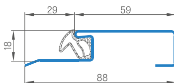
Seuil en tôle inox
