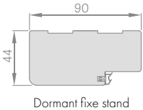
Dormant fixe stand
