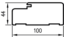
PROFIL OP SOFT
