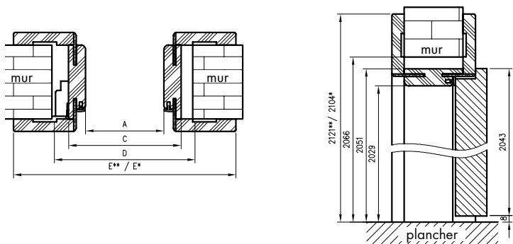
Dimensions pour porte simple vantail
