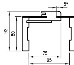
Coupe ORB 075
