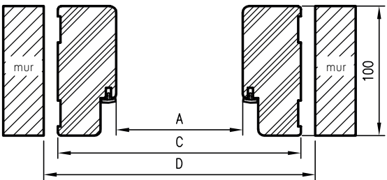
COUPE HORIZONTALE OP
